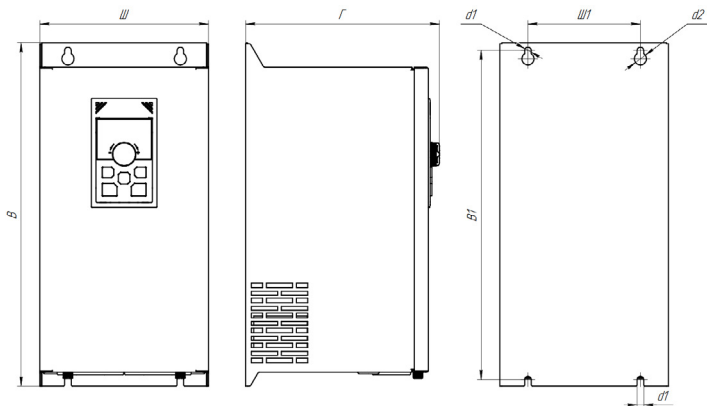
Рис. 2 - Установочные и габаритные размеры тормозного модуля BU, типоразмер 2
